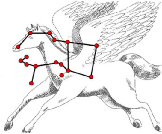
Pegasus:
