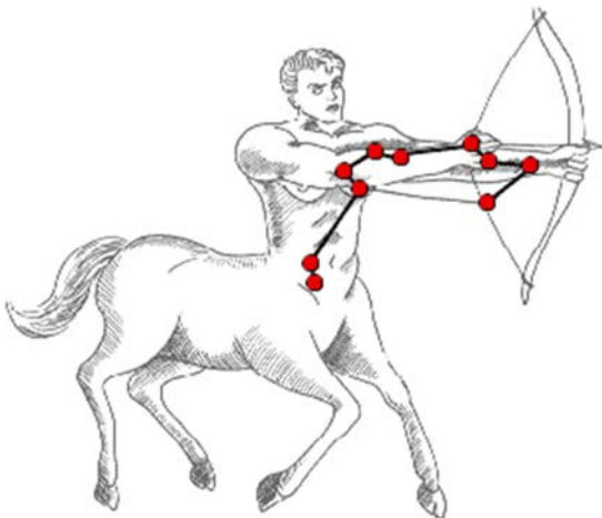
Sagittarius:
