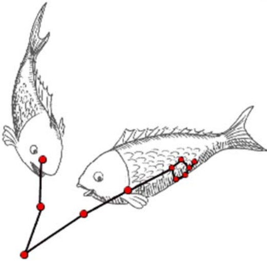
Pisces:
