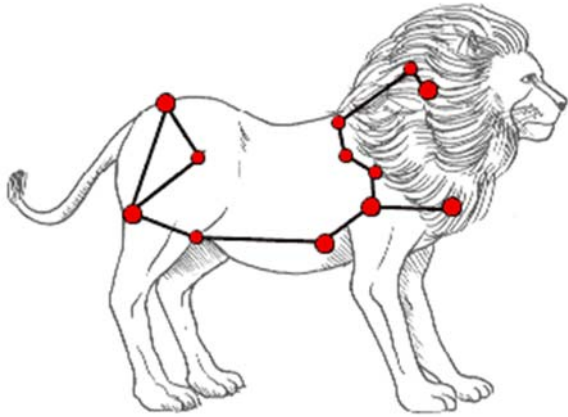
Leo:
