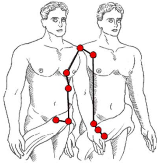
Gemini:
