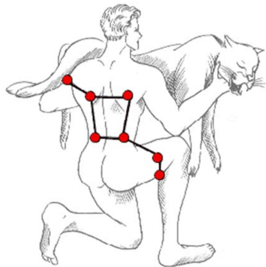
Hercules:
