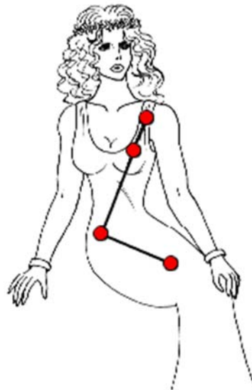
Cassiopeia:
