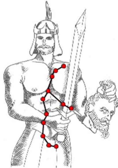
Perseus:
